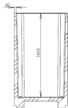
SECTION A-A SCALE 1 : 15
