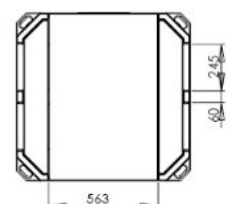
SECTION A-A SCALE 1 : 15
